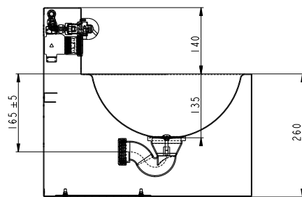
SECCIÓN A-A
