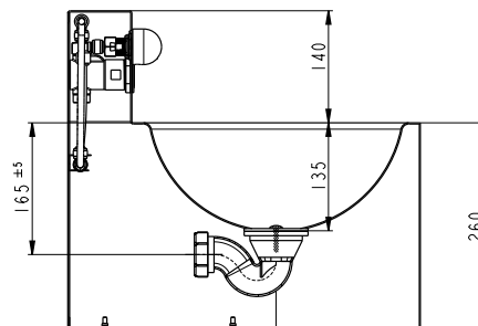
SECCIÓN A-A
