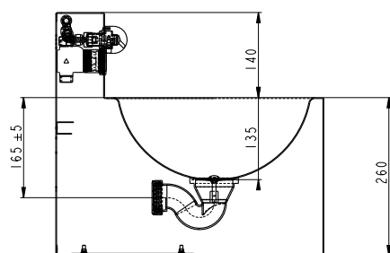
SECCIÓN A-A
